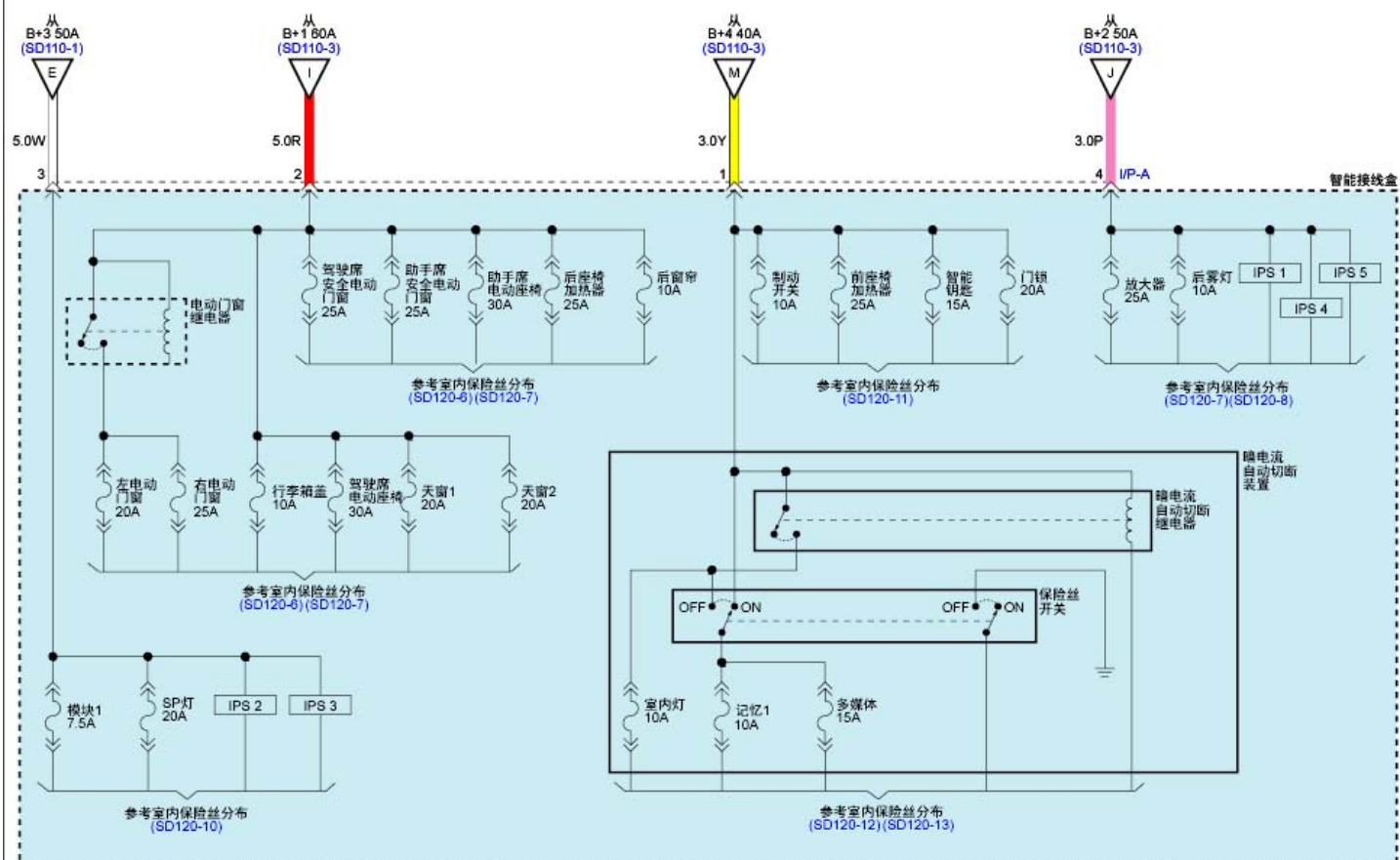
电源分布(13)
